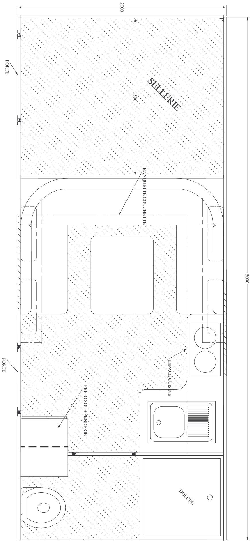
Avant remorque
